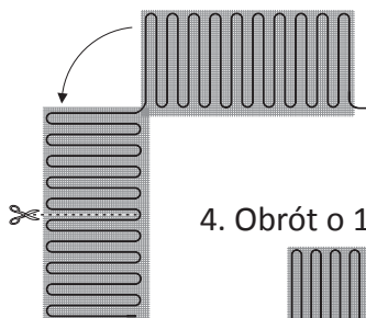
3. Obrót o 90 stopni.
