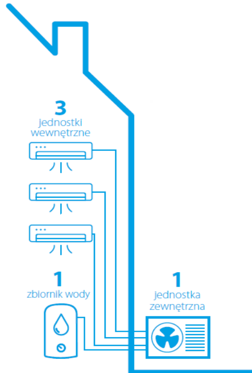
Jednostka zewnętrzna 5MXXM68A9 oraz 5MXXM90A9 Wys. x Szer. x Głęb.: 734 x 1028 x 408 mm
