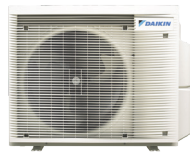
Jednostka zewnętrzna 4MXXM52A9 Wys. x Szer. x Głęb.: 734 x 974 x 401 mm
