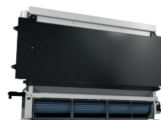
Klimakonwektor FWXM-ATV3(R) Wys. x Szer. x Głęb.: 10: 576 x 725 x 126 mm 15: 576 x 925 x 126 mm 20: 576 x 1125 x 126 mm
