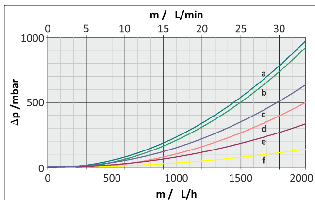
8-5 Krzywa spadku ciśnienia dla wymienników ciepła
