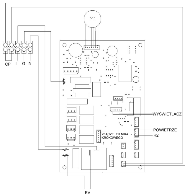
Schemat połączeń
