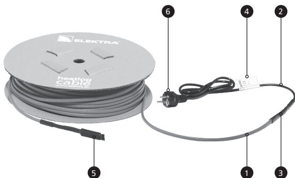
Przewód grzejny ELEKTRA FreezeTec® ready2heat
