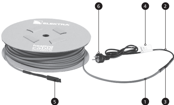
Нагревательный кабель ELEKTRA FreezeTec® ready2heat
