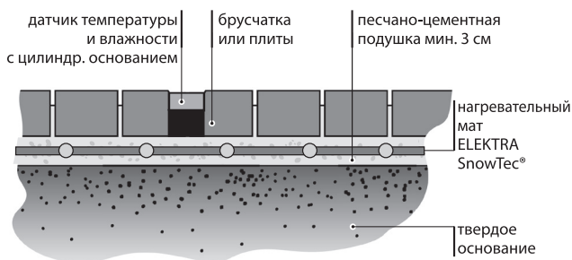
Поперечное сечение тротуара или подъездных путей, с покрытием из плит или брусчатки.
