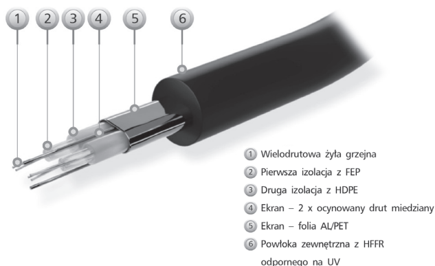
Konstrukcja przewodu grzejnego ELEKTRA TuffTec™
