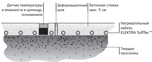
Поперечное сечение тротуара или подъездных путей, изготовленных из бетонной стяжки
