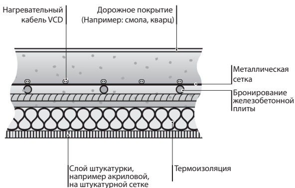
Поперечное сечение подъездного пандуса
