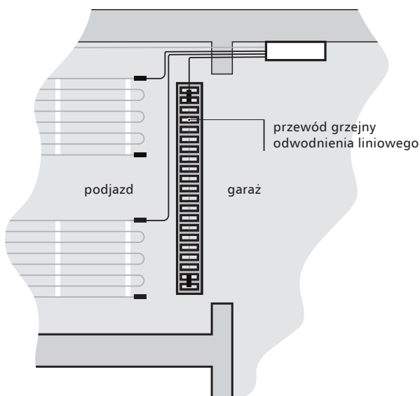
Ogrzewanie odwodnienia liniowego
