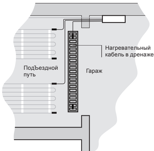
Обогрев линейного дренажа
