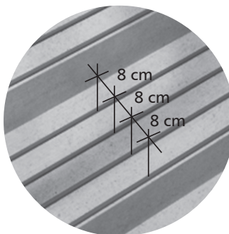
Przykład rozmieszczenia przewodu grzejnego na stopniach schodów
