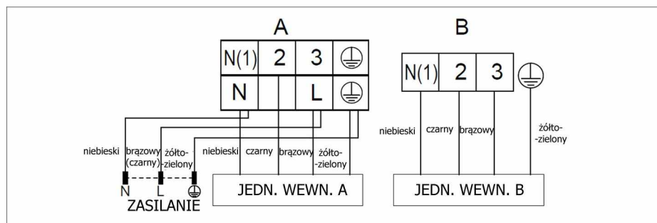
Schemat zasilania
