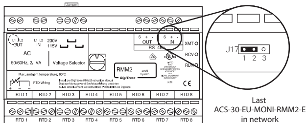
ACS-30-EU-MONI-RMM2-E
